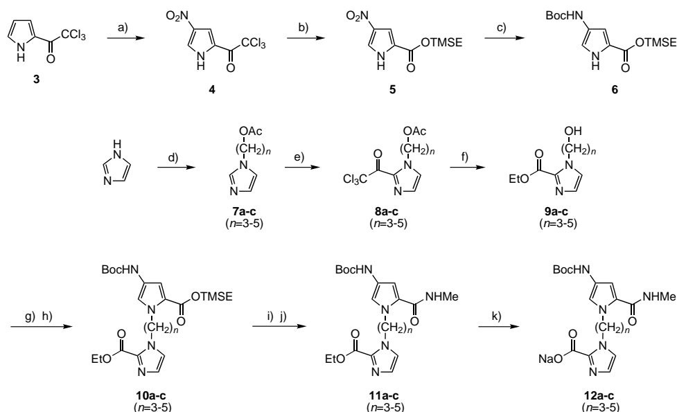
Scheme 1. Synthesis of the U-turn building blocks 12a–c . a) \text{HNO}_3 , \text{Ac}_2\text{O} ; b) TMSEOH, NaH; c) 1. \text{H}_2 , Pd/C, 2. Boc 2 O, NaHCO 3 ; d) \text{Br}(\text{CH}_2)_n\text{OAc} , NaH; e) \text{CCl}_3\text{COCl} ; f) NaOEt; g) 5 , \text{K}_2\text{CO}_3 ; h) 6 , \text{K}_2\text{CO}_3 ; i) TBAF; j) 1. DCC, HOBT, 2. MeNH 2 , DIEA; k) NaOH.
